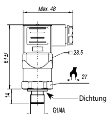
A 10 Druck-Messumformer (Relativdruck, elektrisch Null bei Atmosphärendruck)
